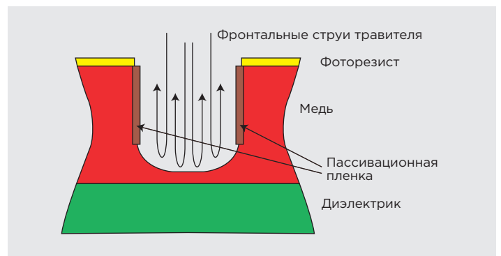
6 Схема движения струй травящего раствора в системе Frezer Style + СЭМАР
