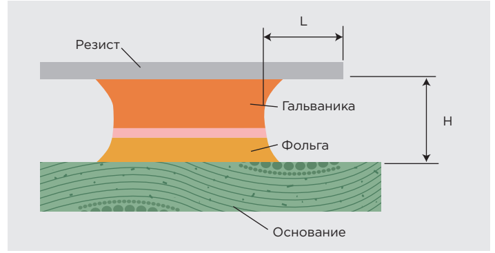
4 Результат изотропного травления меди. Наблюдается боковой подтравивание L печатного проводника
